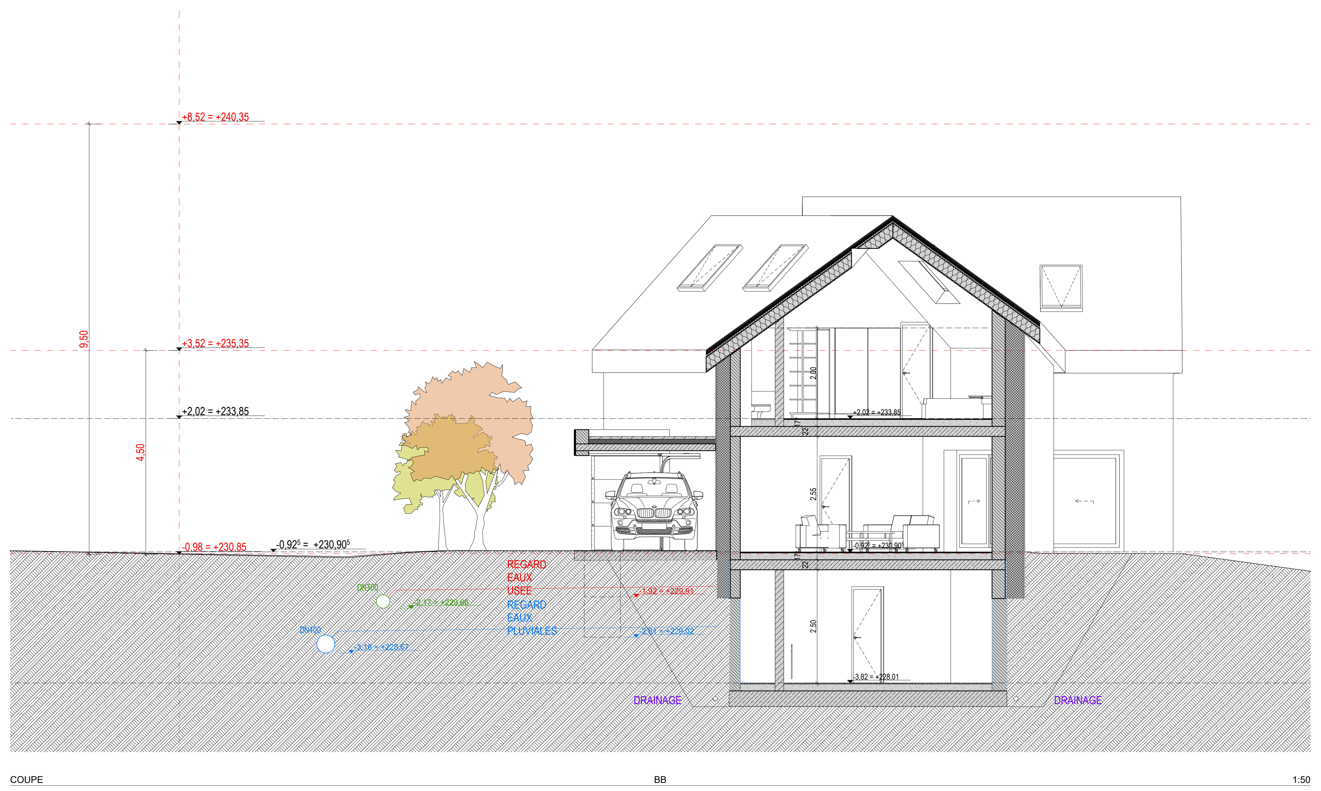
COUPE BB 1:50
