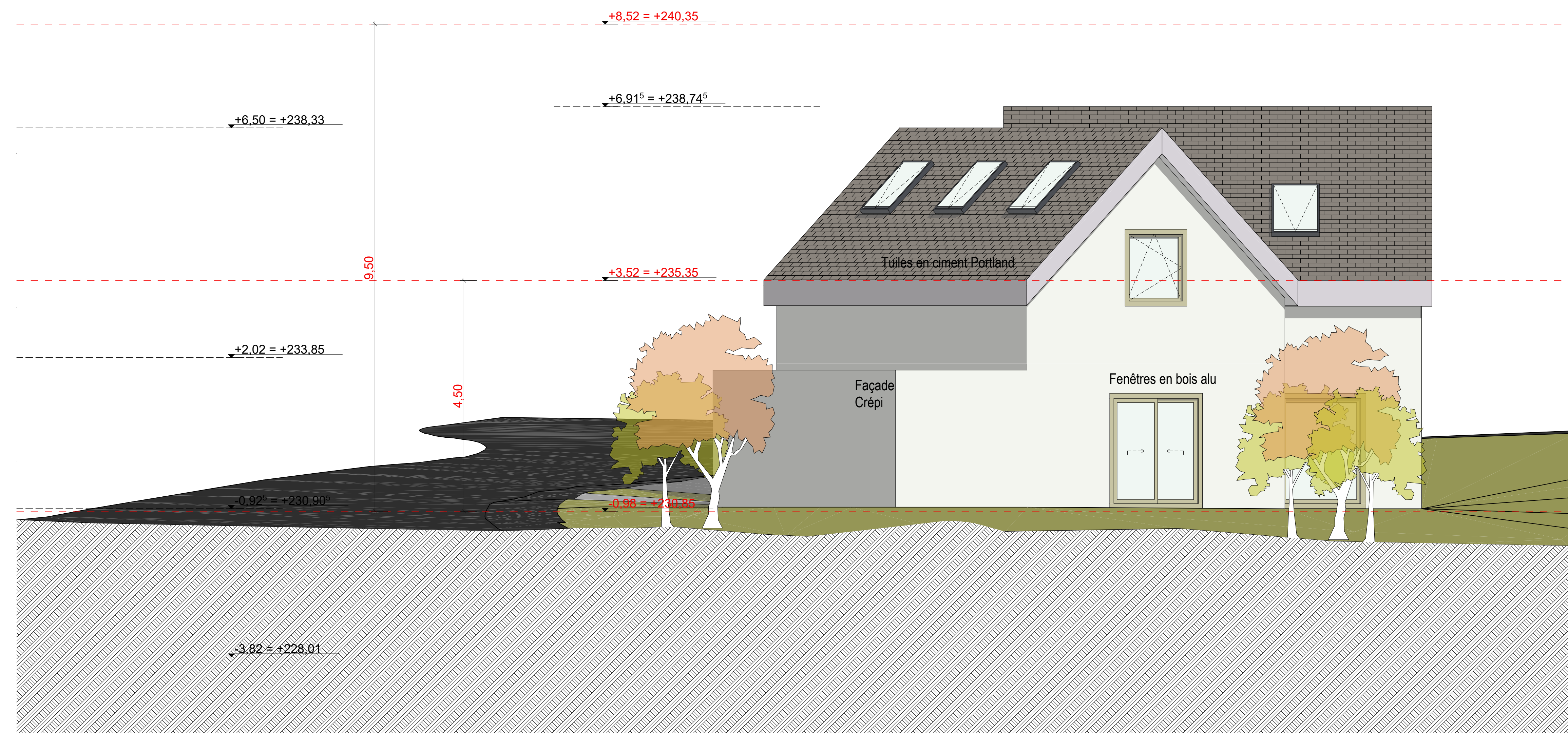
Façade nord-est 1:50
