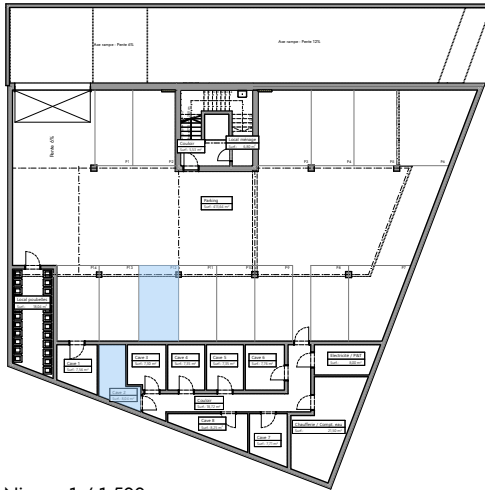
Niveau -1 / 1:500
